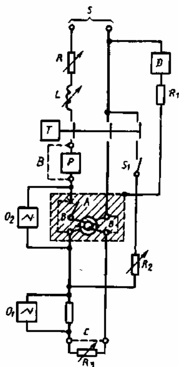
Рисунок 5 — Схема испытательной цепи для проверки правильности координации с аппаратом защиты от коротких замыканий и номинальной включающей и отключающей способностью однополюсного УЗО — D с двумя токопроводящими путями в однофазной цепи и без встроенной защиты от коротких замыканий
