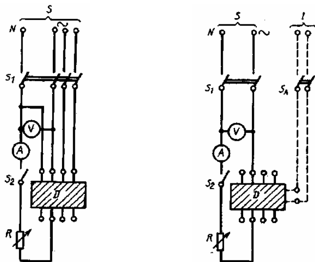
S — источник электрической энергии; I — независимая линия электропитания; V — вольтметр; A — амперметр; S_1 — многополюсный выключатель; S_2 — однополюсный выключатель; D — испытуемое УЗО — Д; R — регулируемый резистор; S_A — дополнительный выключатель
