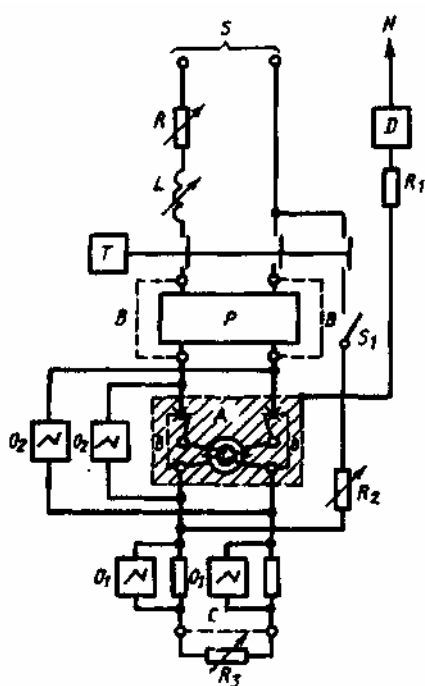
Рисунок 6 — Схема испытательной цепи для проверки правильной координации с аппаратом защиты от коротких замыканий и номинальной включающей и отключающей способностью двухполюсного УЗО — D без встроенной защиты от коротких замыканий в однофазной цепи
